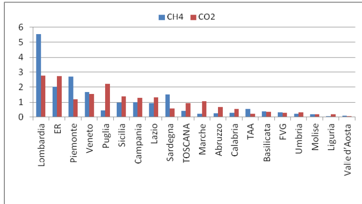
Fonte: Elaborazioni su dati Inventario Nazionale delle Emissioni 2005 e ENEA(2010)
