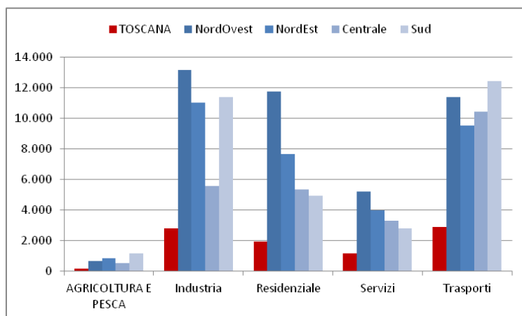
Fonte: Elaborazioni su stime ENEA
